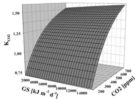
Abbildung 1: K CO 2 in Abhängigkeit von CO 2 -Konzentration der Atmosphäre und Globalstrahlung
