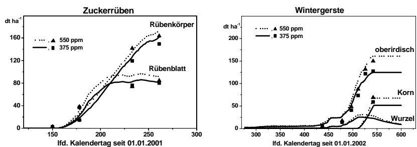
Abbildung 2: Dynamik einzelner Biomassefraktionen für Zuckerrüben (2001) und Wintergerste (2002/2003) bei CO 2 -Konzentrationen der Atmosphäre von 375 ppm und 550 ppm, berechnet mit AGROSIM-Modellen und verglichen mit Messdaten aus dem FACE-Experiment
