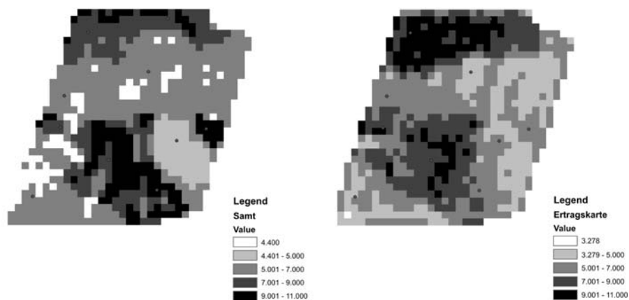
Abbildung 1: Vergleich zwischen der mit Hilfe der in SAMT integrierten Methodik erstellten Ertragskartierungskarte (links) und der für den Schlag aus Mährescherdaten generierten Ertragskarte (rechts)
