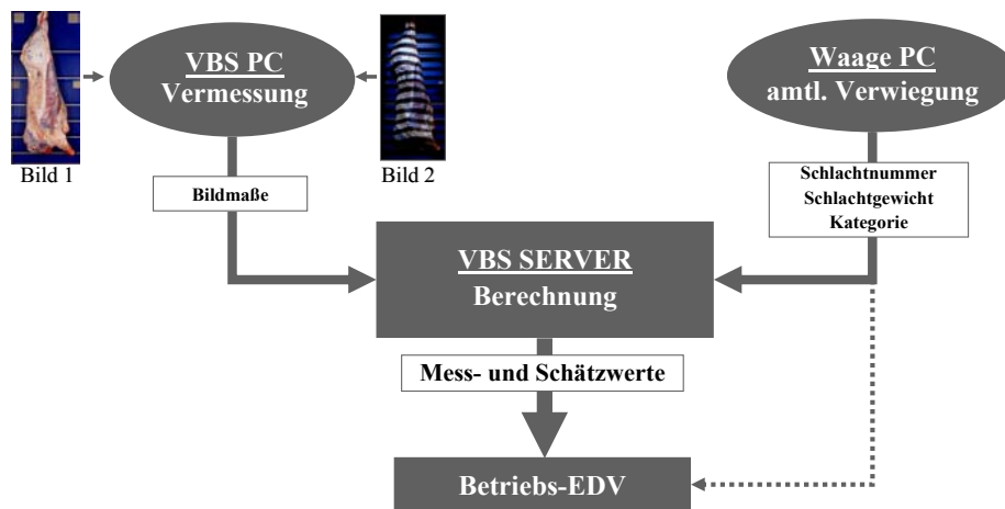
Abbildung 1: Funktionsweise des VBS 2000 (eigene Darstellung)
