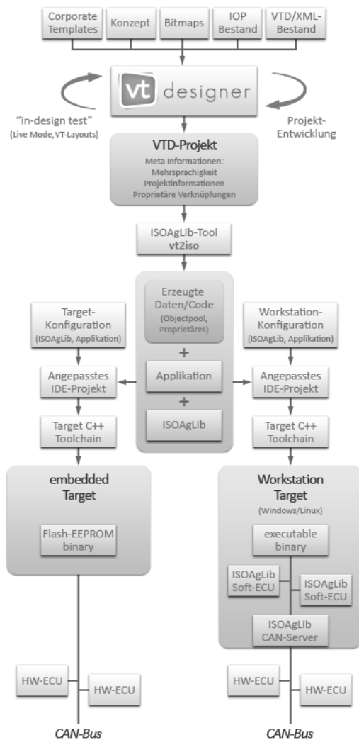
Abbildung 2: ISOAgLib-Toolchain (eigene Darstellung)
