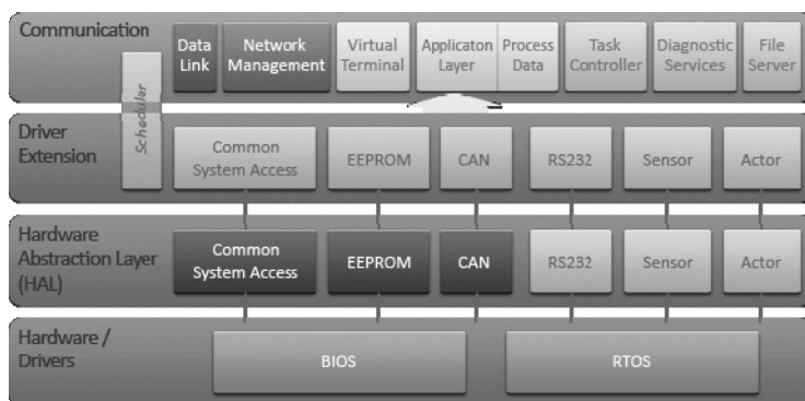
Abbildung 1: Modul- und Schichtenarchitektur der ISOAgLib-Software (eigene Darstellung)
