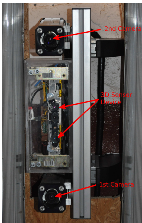
Abbildung 1: Bilderfassungs-System
