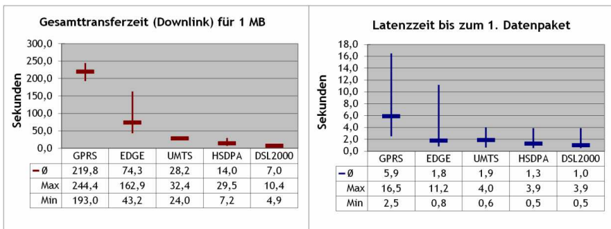
Abb. 2: Empirische Ergebnisse zur Datenfunk-Performance gegliedert nach Übertragungstechnik.
