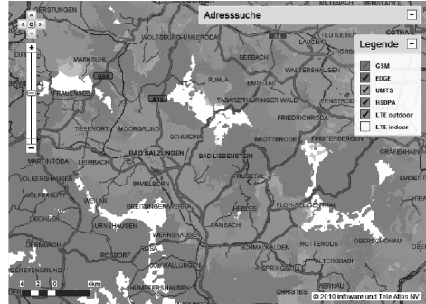
Abbildung 1: Beispielhafte ländliche Netzabdeckungskarte mit Versorgungslücken (weiße Flächen) 2
