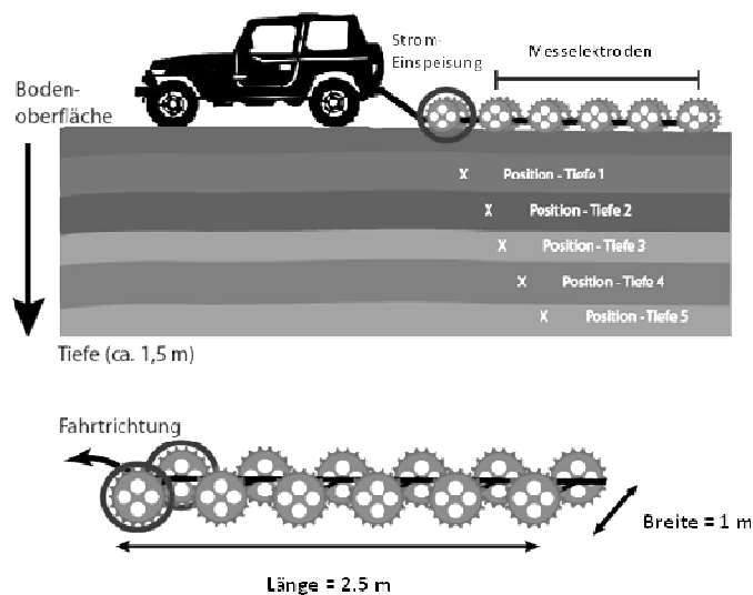
Abb. 1: Der ER Sensor – bestehend aus der Stromeinspeisung (1. Achse) und den Messdipolen (2.-6. Achse)
