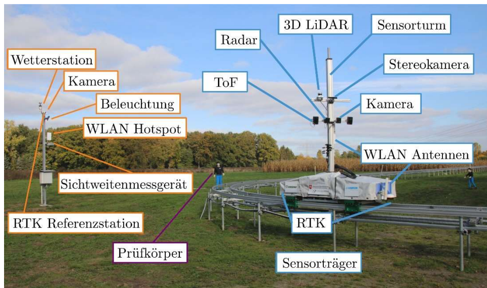
Abb. 2: Die zu evaluierende Sensorik wird auf dem drehbaren Sensorturm befestigt. Auf dem Testfeld steht ein Mast, an dem die Hardware zur Überwachung und Kommunikation mit dem Dolly befestigt ist.
